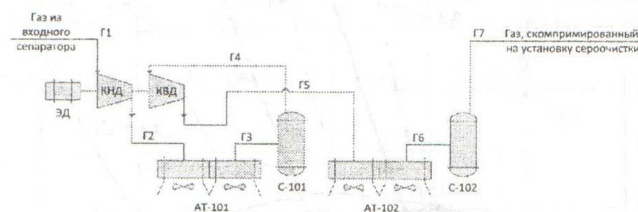
Рис. 1 – Технологическая схема КС
